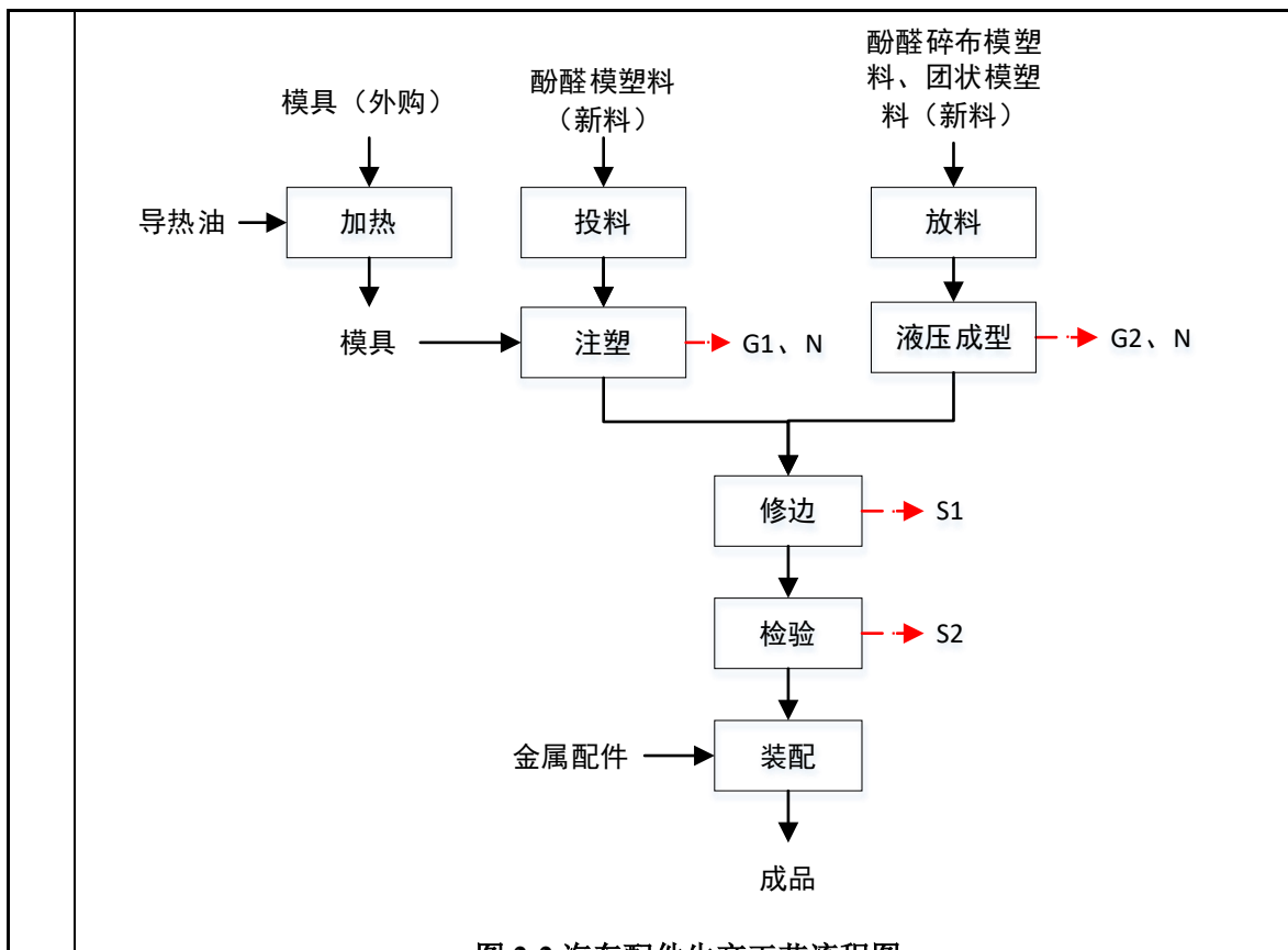
图 2-2 汽车配件生产工艺流程图
